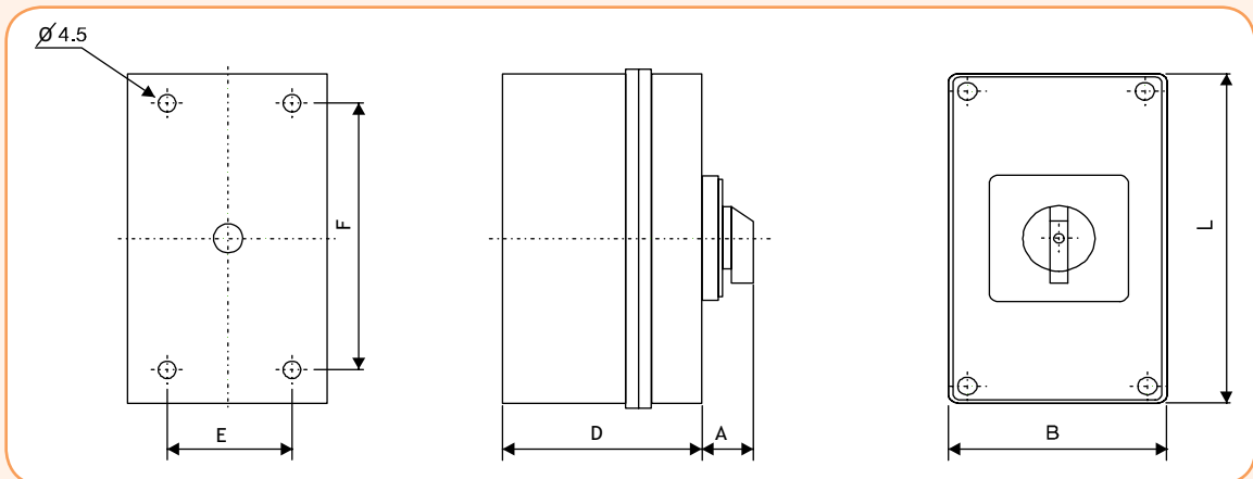
Размещение отверстий
