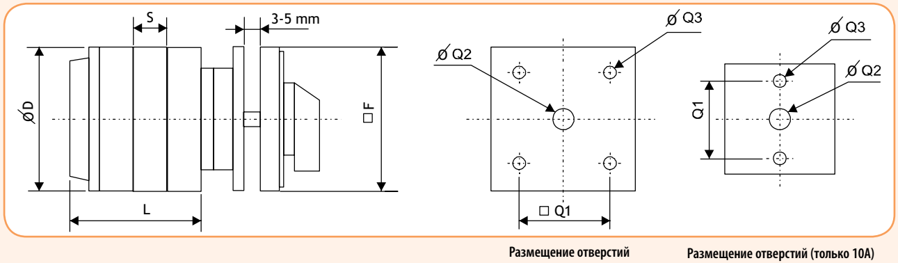
Размещение отверстий
